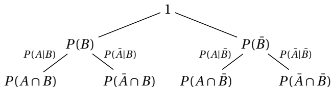
Abbildung 9: Zweistufiger Entscheidungsbaum.
