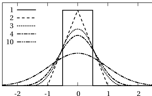
Abbildung 22: Dichtefunktion der Summe von 1, 2, 3, 4 und 10 unabhängigen Zufallsvariablen mit der Gleichverteilung zwischen -0.5 und 0.5 .
