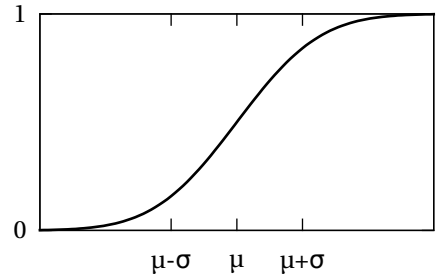
(b) Verteilungsfunktion
