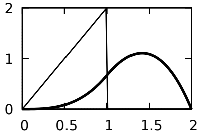
Abbildung 21: Dichtefunktionen f_X(x) = f_Y(x) = 2x und f_{X+Y}
