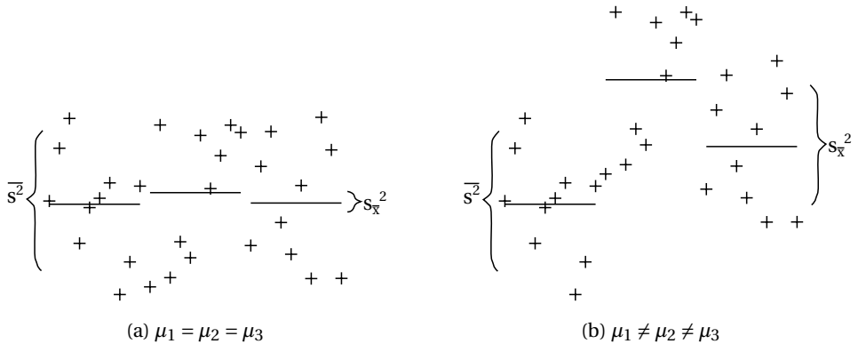
Abbildung 25: Mittelwert der Varianzen und Varianz der Mittelwerte bei ANOVA.
