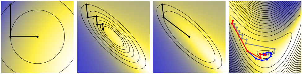
(a) Orthogonale Richtungen für A = I : \mathbf{x}^T A \mathbf{x} = \mathbf{x}^T \mathbf{x} (b) Orthogonale Richtungen für A nicht-diagonal (c) Konjugierte Richtungen (d) Nicht-quadratische Funktion f . Grau: normaler Gradient-Descent, blau: Fletcher-Reeves, rot: Polak-Ribière.
