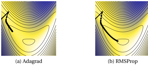
Abbildung 9: Gradient-Descent mit Koordinaten-adaptiven Lernraten
