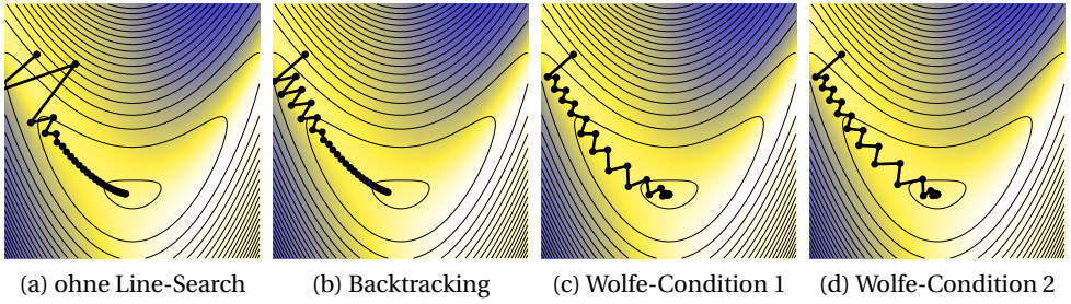
Abbildung 8: Gradient-Descent
