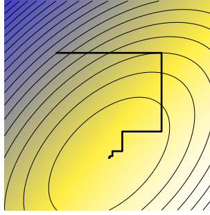
Abbildung 2: Coordinate-Descent
