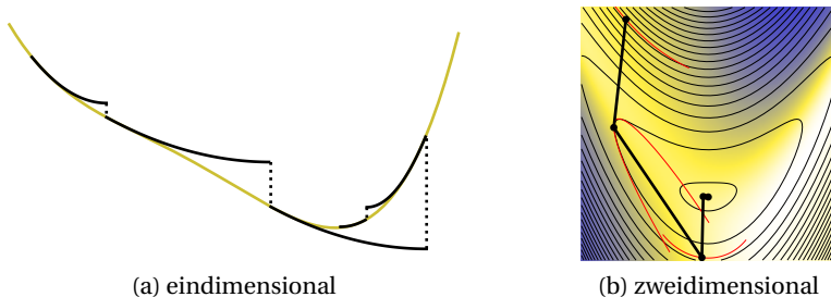
Abbildung 13: Newton-Methode
