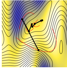
(b) Levenberg-Marquard
